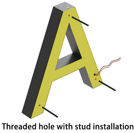
2.Stud Installation
